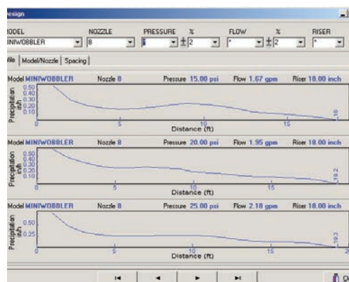
Les profils d'arroseur illustrent la quantité d'eau qui serait distribuée à différents intervalles ainsi que le rayon de projection (portée).
