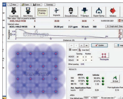
Les densogrammes illustrent l'uniformité, le diamètre ainsi que la surface d'arrosage d'un profil donné.
